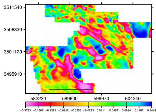
IP 090Hz DT
