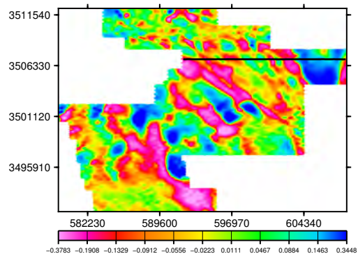
IP 090Hz DT
